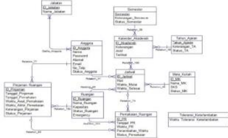
Gambar 6. Bentuk Relasi Pusat Data
