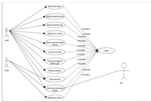
Gambar 1. Use Case Diagram Aplikasi
