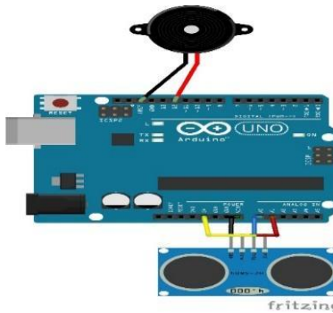
Fig 4. Tool Schematic Suite
